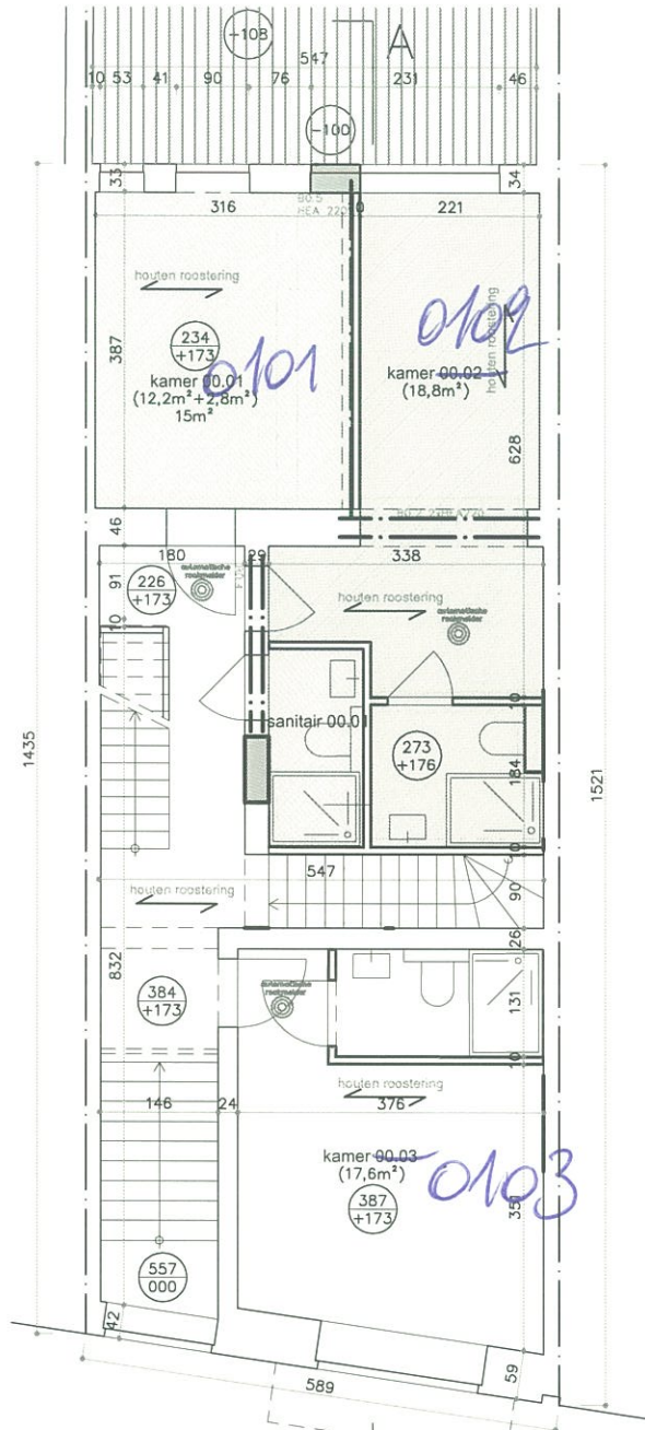
GELIJKVLOERS A
